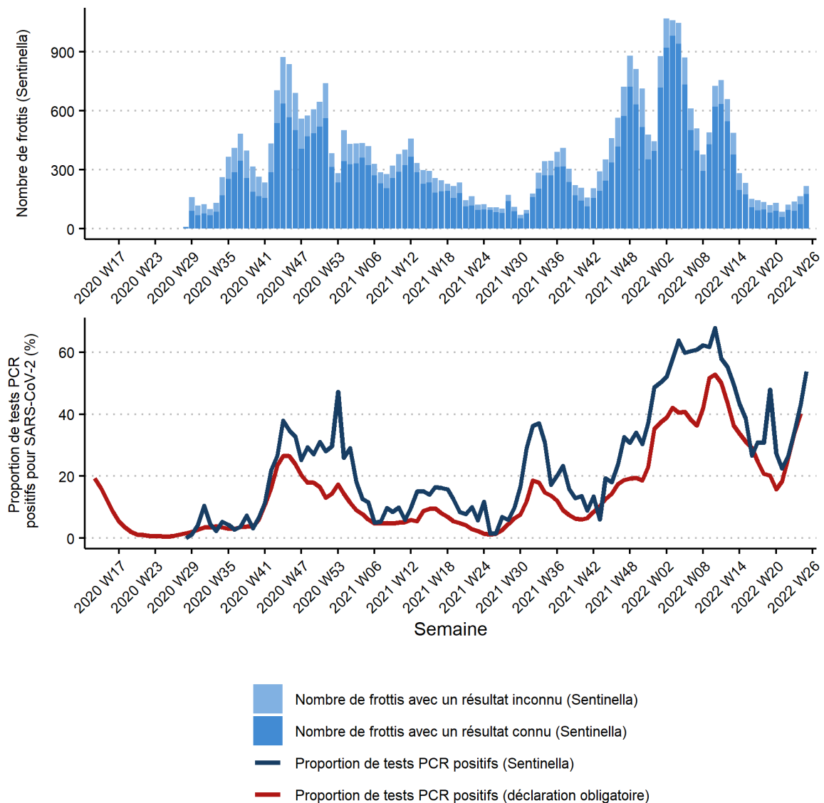
Figure 2. Nombre de patients avec une suspicion de COVID-19 chez lesquels un frottis a été effectué (graphique du haut) et la proportion de tests PCR positifs pour le SARS-CoV-2 (graphique du bas). Ces informations sont déclarées depuis la semaine 29/2020. À titre de comparaison, la proportion de tests PCR positifs enregistrés dans le cadre du système de déclaration obligatoire est également indiquée.
