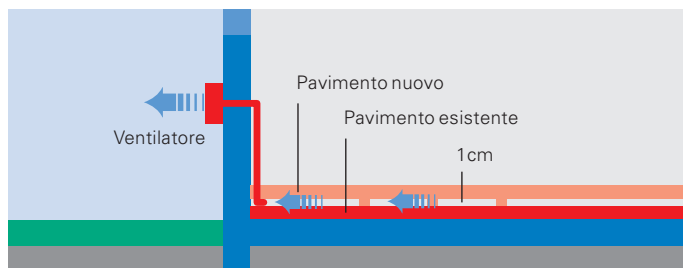
Aspirazione da intercapedine in un locale singolo.
