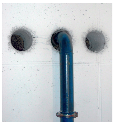
Grandi aperture e fessure nelle parti dell'edificio a contatto col terreno devono essere sigillate.
