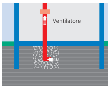
Aspirazione puntuale dal terreno con evacuazione dell'aria sul tetto.
