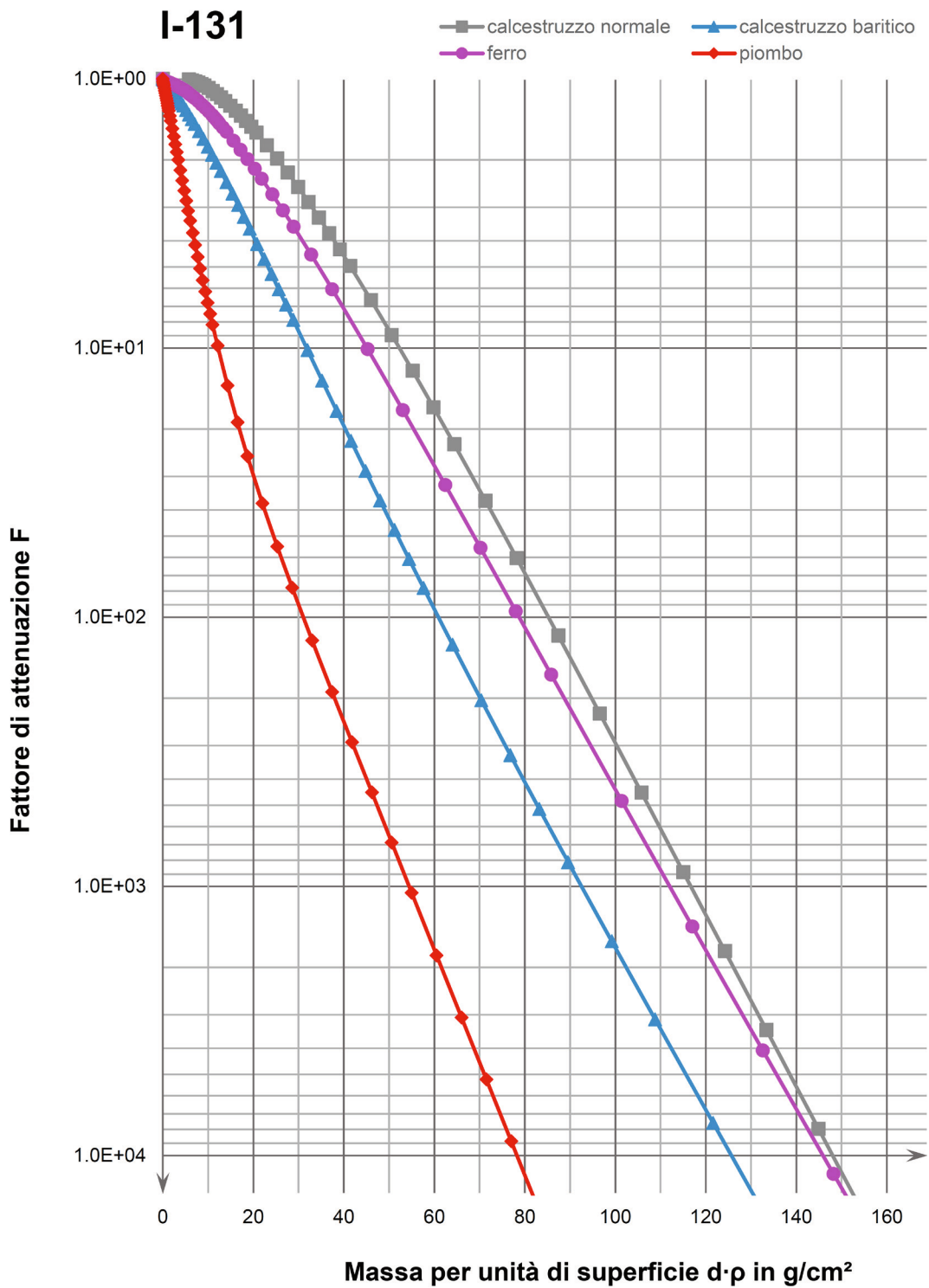
Figura A1 Fattori di attenuazione F per I-131 in funzione della massa per unità di superficie del materiale di schermatura d \cdot \rho in g/cm^3
