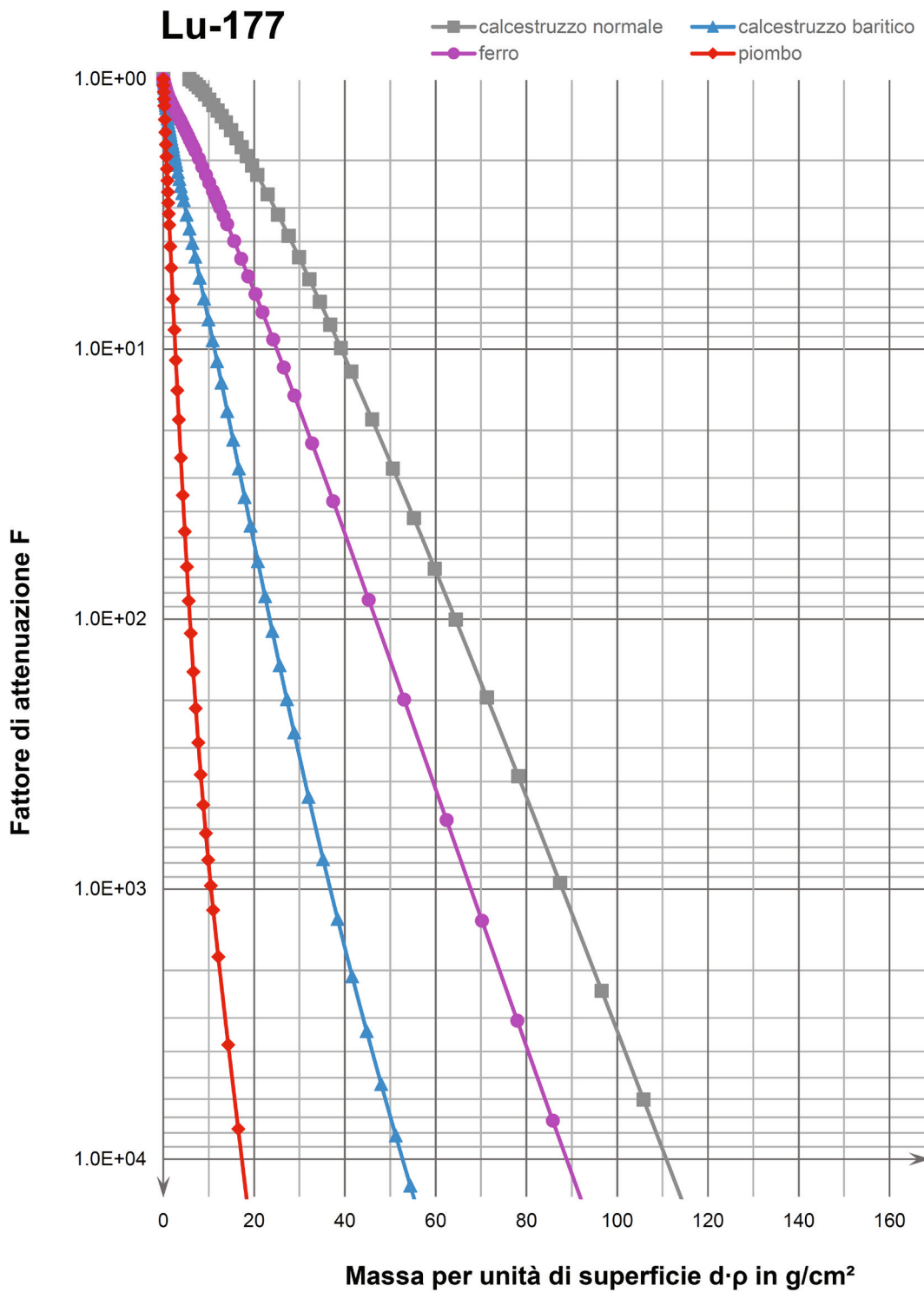
Figura A2 Fattori di attenuazione F per Lu-177 in funzione della massa per unità di superficie d \cdot \rho in g/cm^2
