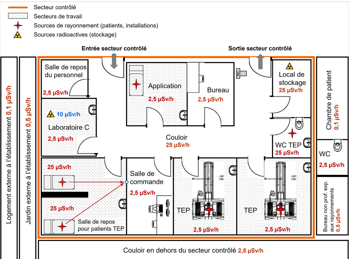
Figure 1 Exemple de plan d'un secteur contrôlé avec les valeurs directrices pour les débits de dose ambiante dans les différents locaux. Les valeurs en rouge se réfèrent au débit de dose dû aux sources présentes dans les locaux adjacents. La valeur en bleu correspond à la valeur directrice concernant les sources stockées dans le laboratoire C.
